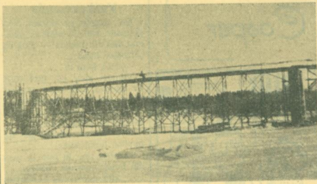
Bropelarna till nya bron över Öreälven är klara. Nu återstår överförandet av stålkonstruktionen. Hammarbyverken står som leverantör.
