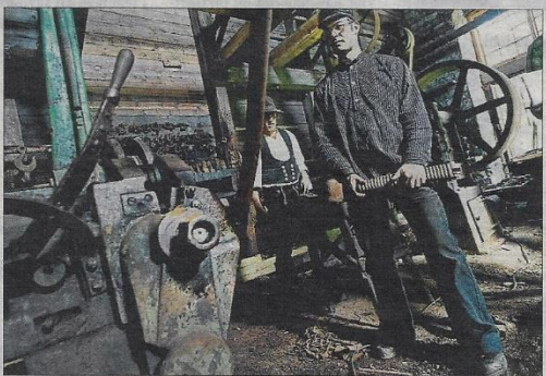
Bockningsmaskinen fungerar efter att ha stått stilla i 60 år.
